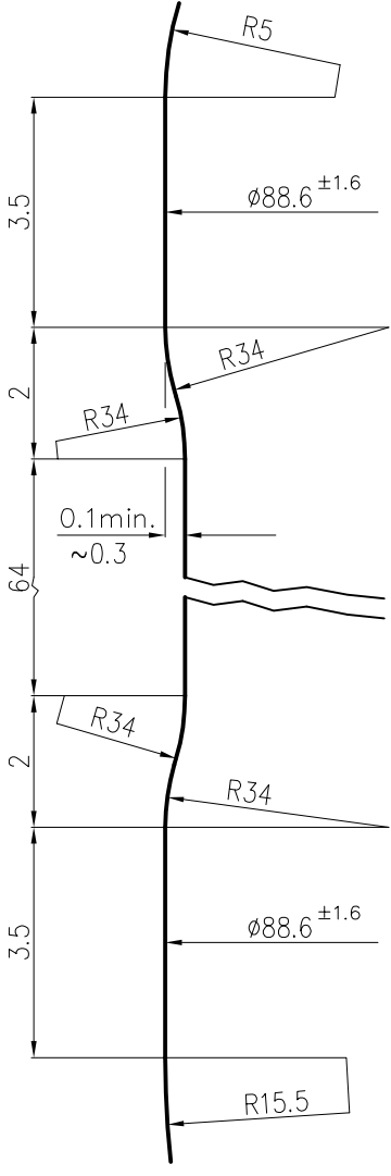
ETİKET GİRİNTİ DETAYI
