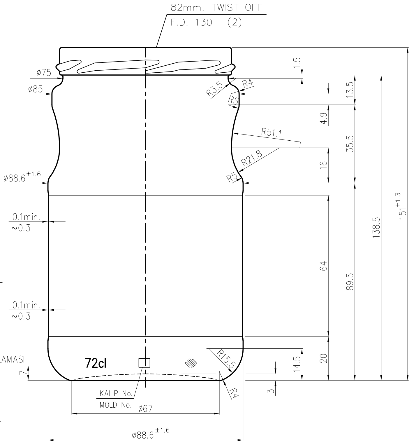
ETİKET GİRİNTİ DETAYI
